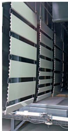
Bei Angelier- und Einbrennofen reduziert eine Doppelschleuse den Wärmeverlust, sodass die Türen nur bei speziellen Anforderungen geschlossen werden müssen.
